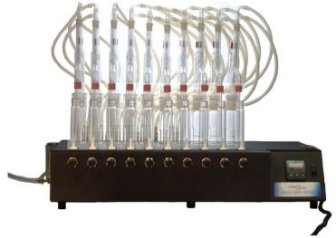
Bộ chưng cất Ammonia/ Phenol 10 vị trí Midi-Vap 4000
